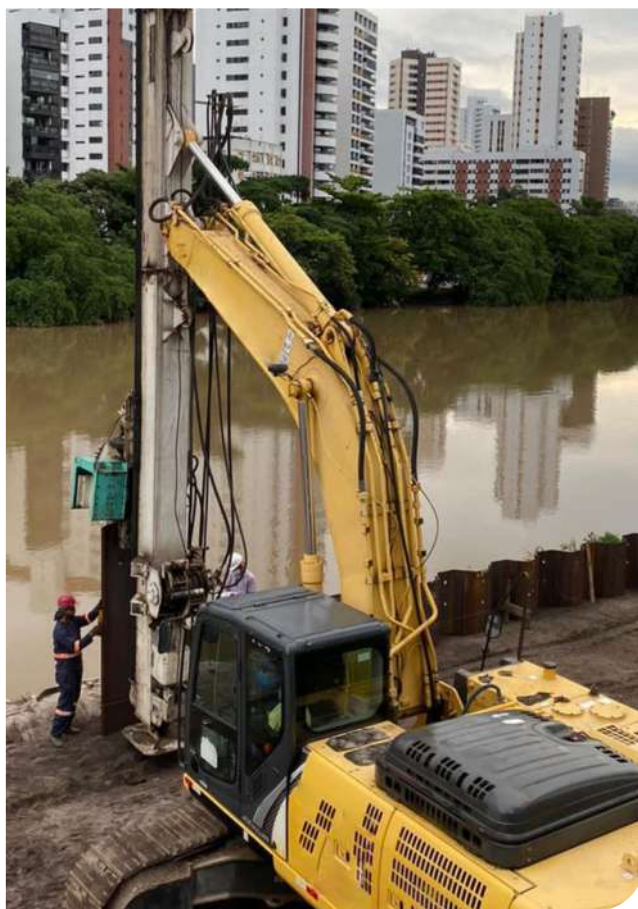
Martelo vibratório montado em equipamento com torre guia Local: Rio Capibaribe, PE
