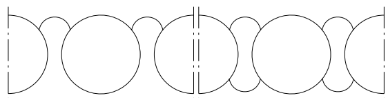
Células circulares com estacas de junção de 35°
